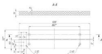
Рис. 2. Размеры бруса. * – размер определяется по месту.
