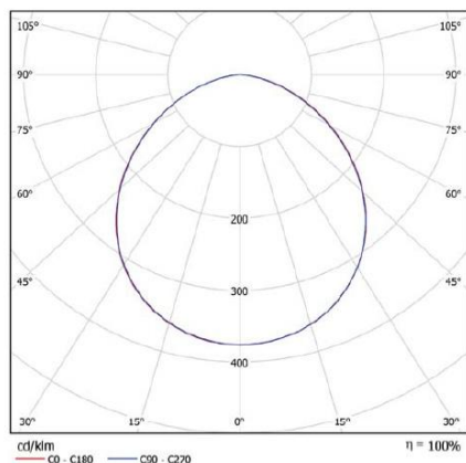
Световые конические пучки
