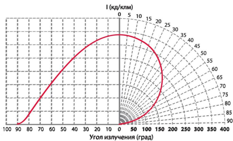
Кривые силы света
